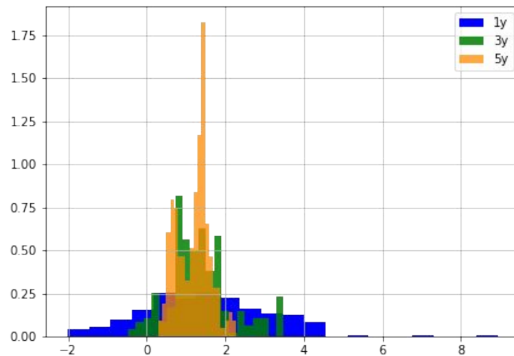
Histogram Sharpe ratia pro 1,3 a 5 leté posouvající se časové okno.
