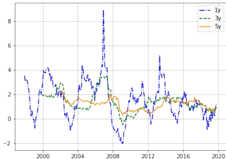
Sharpe ratio strategie pro 1,3 a 5 leté posouvající se časové okno.
